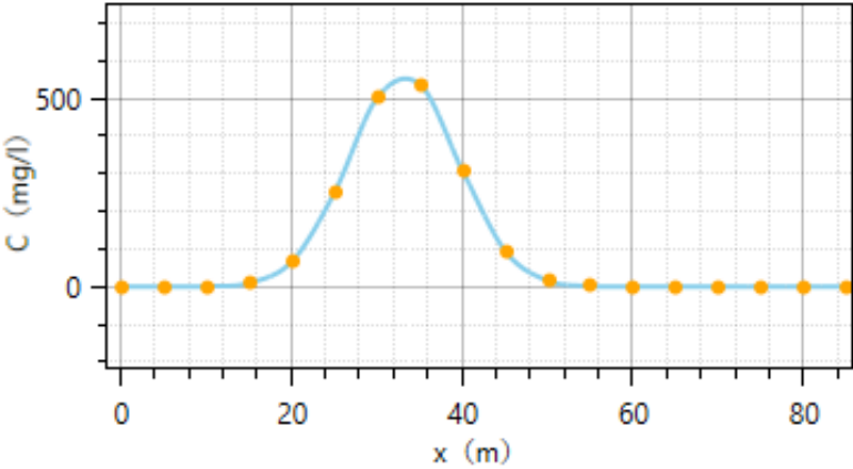
图 6.3-2（1）柴油储罐破损渗漏 100 天石油类污染物不同距离浓度预测曲线
