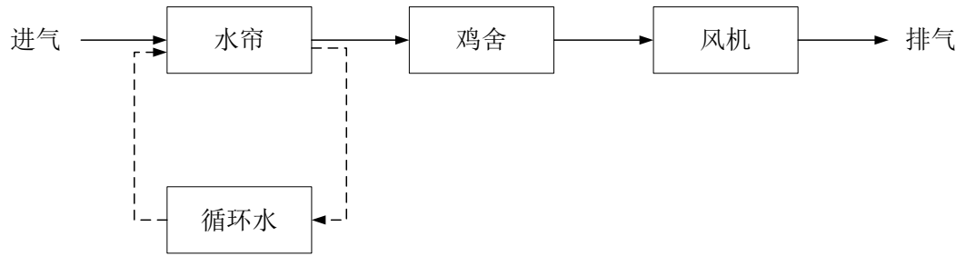
图 3.1-3 湿帘通风系统示意图
