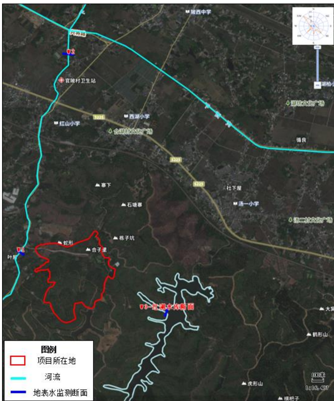
图 4.2-4 地表水及地下水监测布点图
