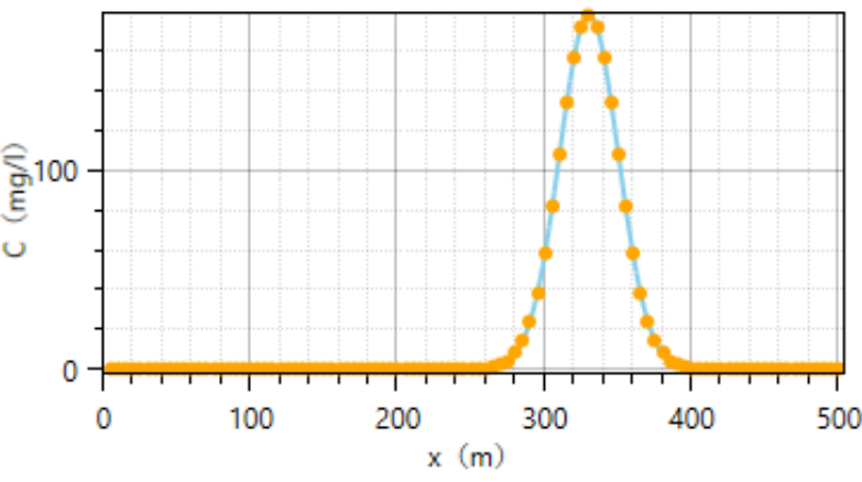
图 6.3-2（2）储罐破损渗漏 1000 天石油类污染物不同距离浓度预测曲线
